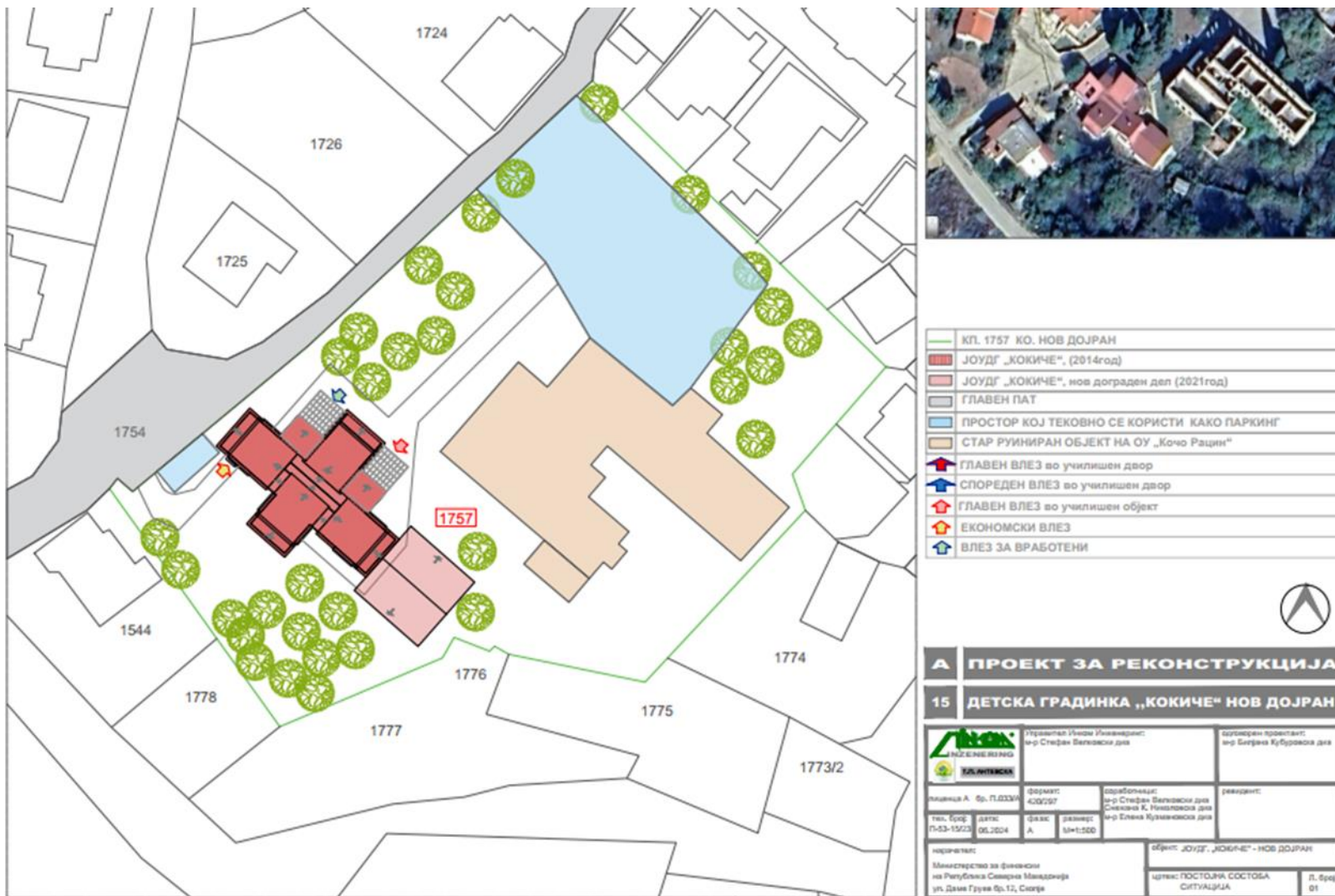
Слика: Индикативна шема на градилиште (шематски приказ)
